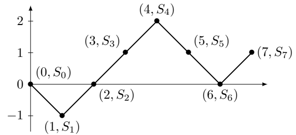
Figure 1 Un chemin de longueur 7
